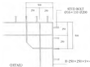
〈DETAIL〉
