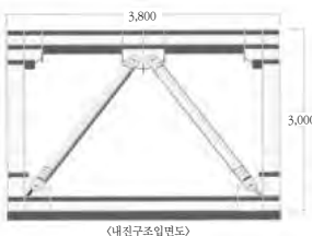
〈내진구조입면도〉
