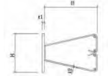
〈ACT PILE〉
